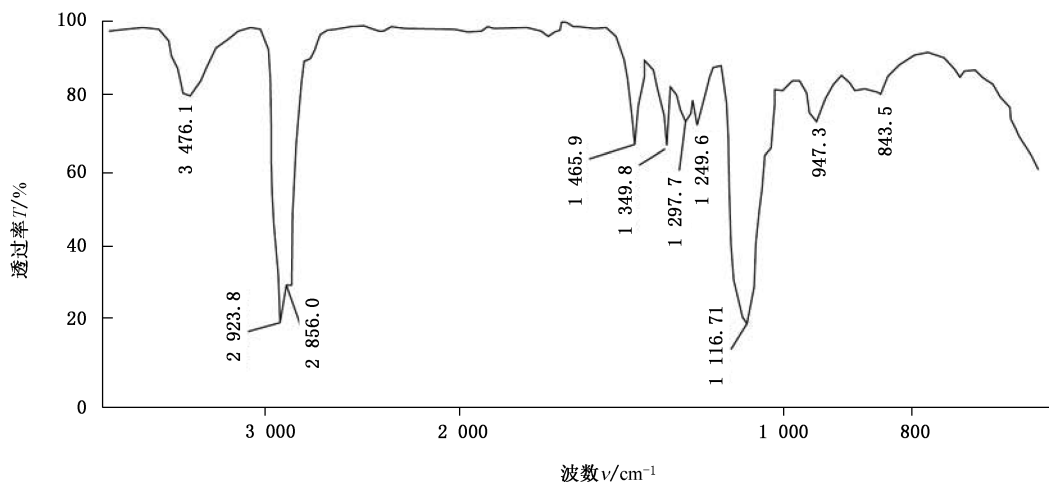
图 C.1 聚氧乙烯脂肪醇醚-8 的红外光谱图
